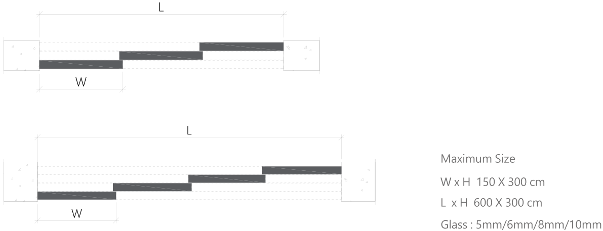
Horizontal section 水平剖面圖
