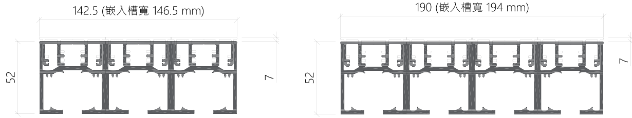
Top Rail specification / Panel profile specification 上軌道規格 / 薄框型材規格
