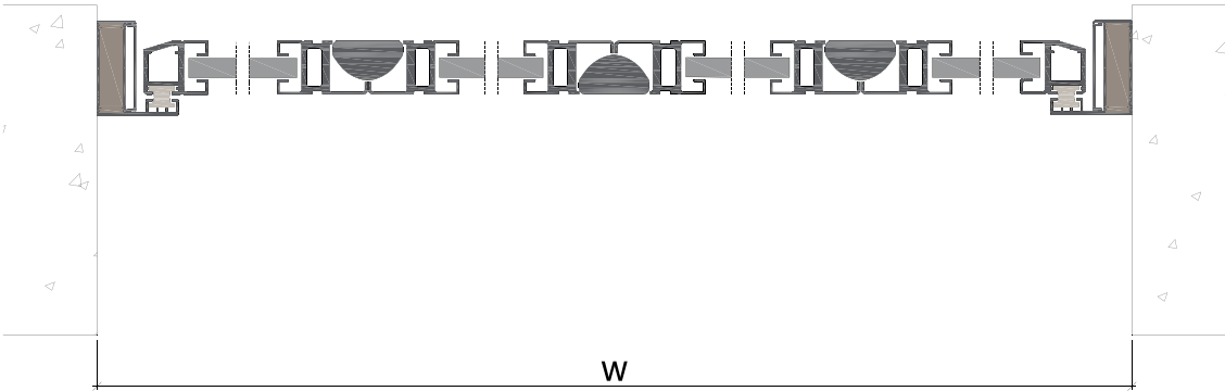
Horizontal section 水平剖面圖
