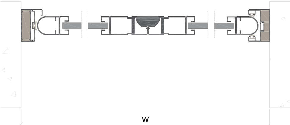
Horizontal section 水平剖面圖
