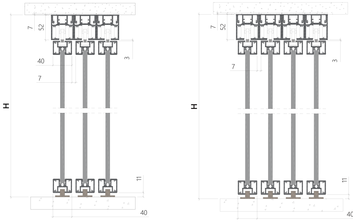
Top Rail specification / Panel profile specification 上軌道規格 / 薄框型材規格
