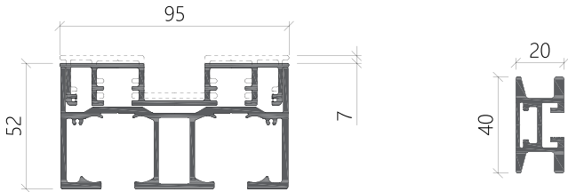
Top Rail specification / Panel profile specification 上軌道規格 / 薄框型材規格
