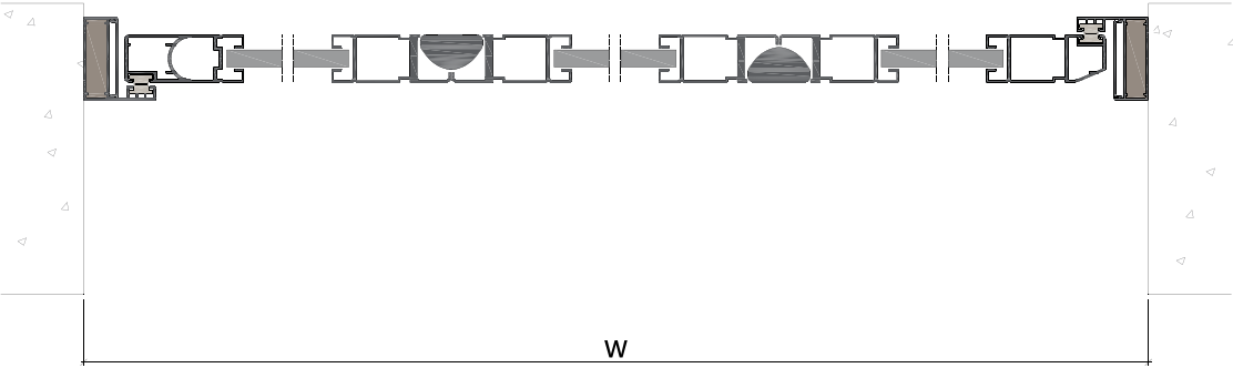
Horizontal section 水平剖面圖
