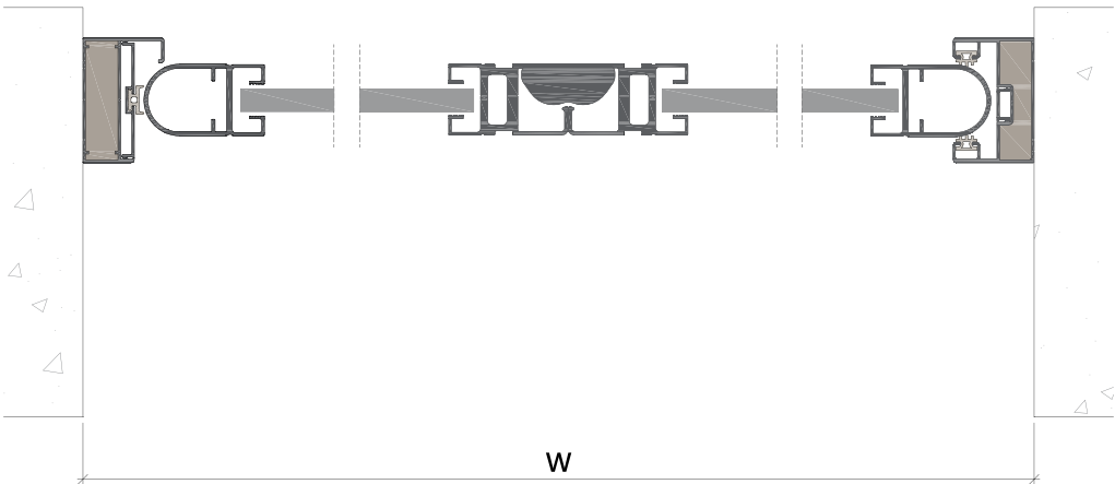
Horizontal section 水平剖面圖
