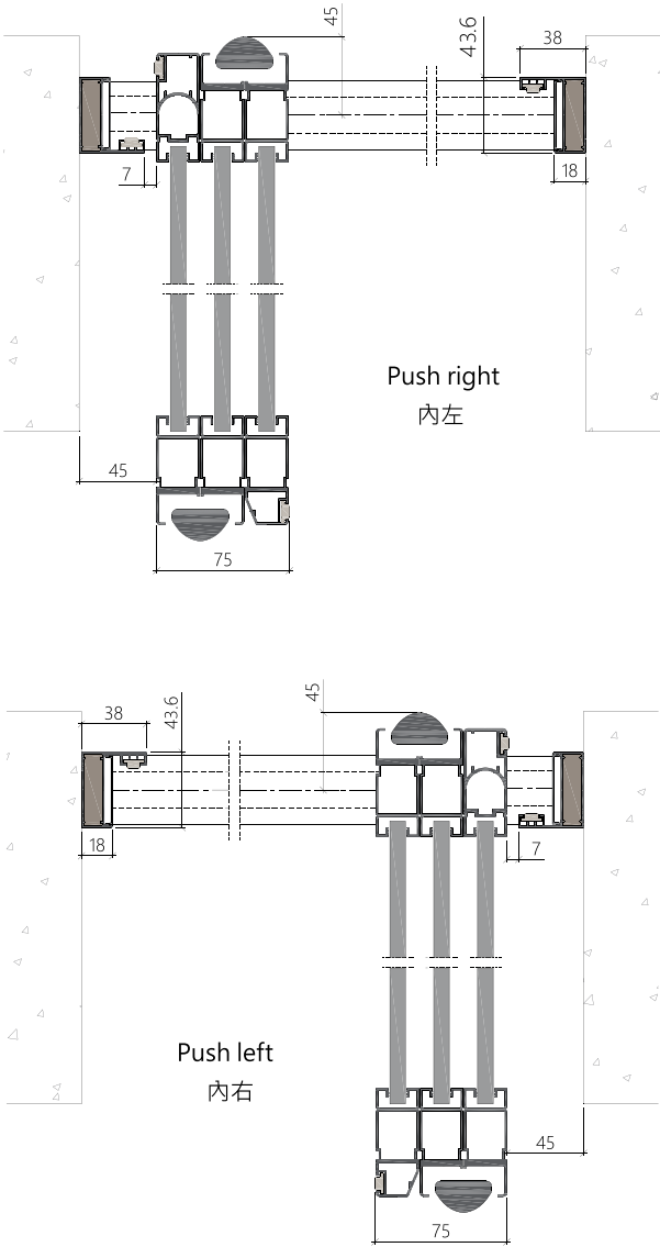
Horizontal section 水平剖面圖
