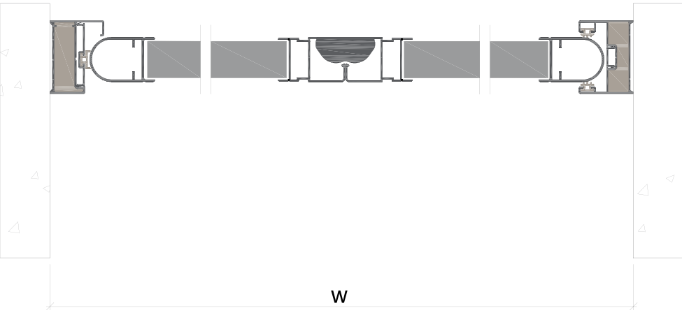
Horizontal section 水平剖面圖
