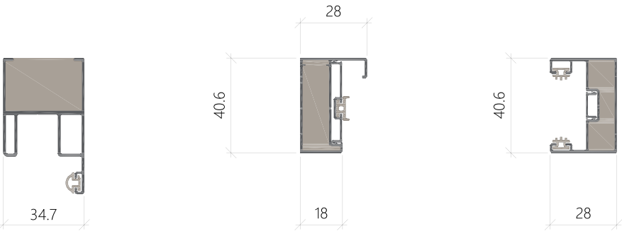
Horizontal section 水平剖面圖
