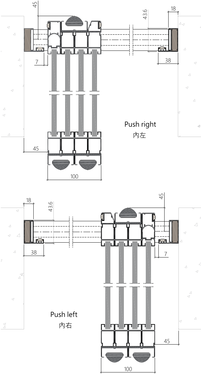
Horizontal section 水平剖面圖
