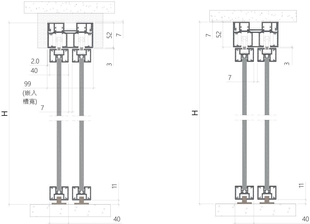
Top Rail specification / Panel profile specification 上軌道規格 / 薄框型材規格
